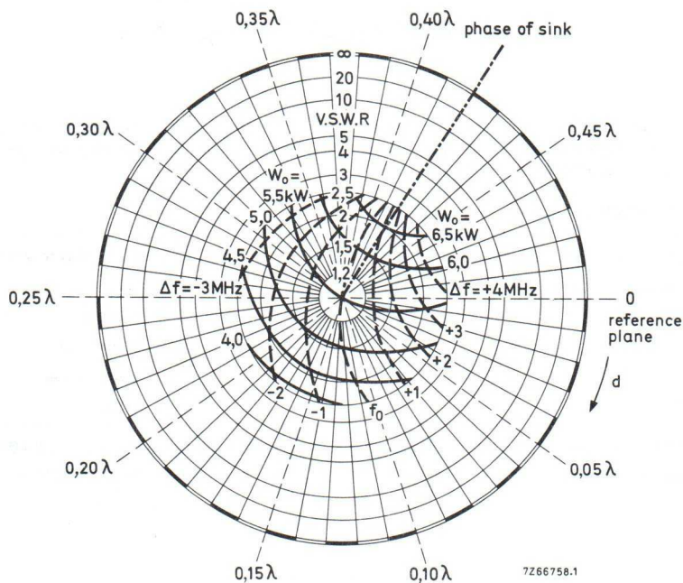
Fig. 16 Load diagram.
