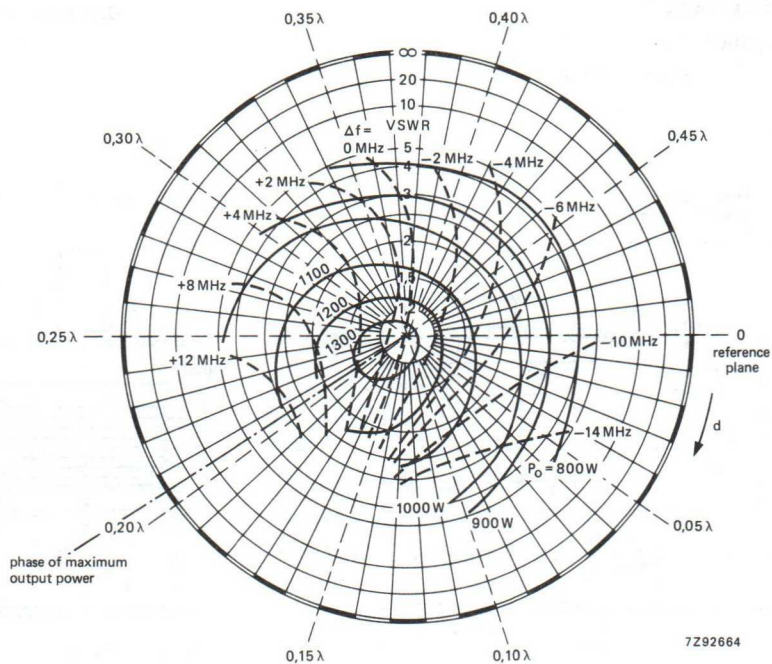
Fig. 4 Load diagram.
