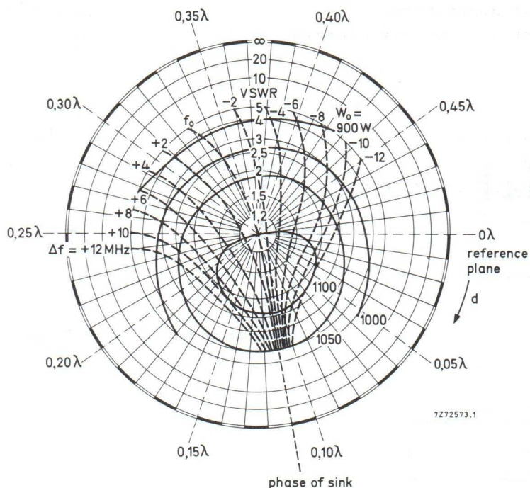
Fig. 5 Load diagram.
