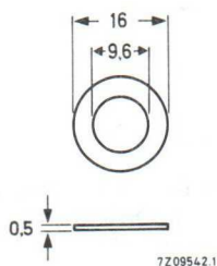
Fig. 4 Washer type 55328.
