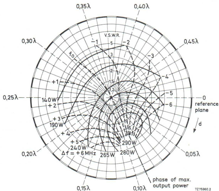
Fig. 3 Load diagram.
