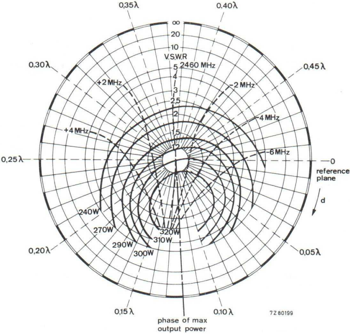
Fig. 3 Load diagram.
