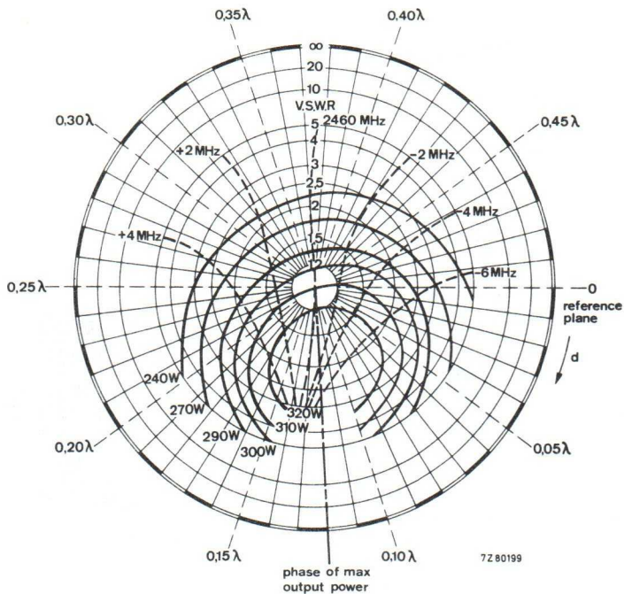
Fig. 4 Load diagram.
