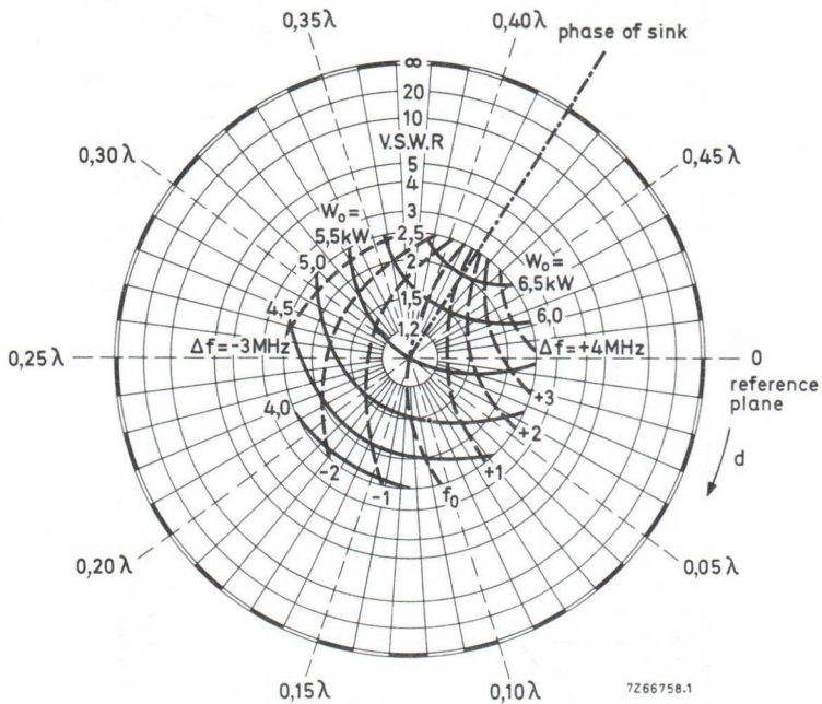
Fig. 16 Load diagram.
