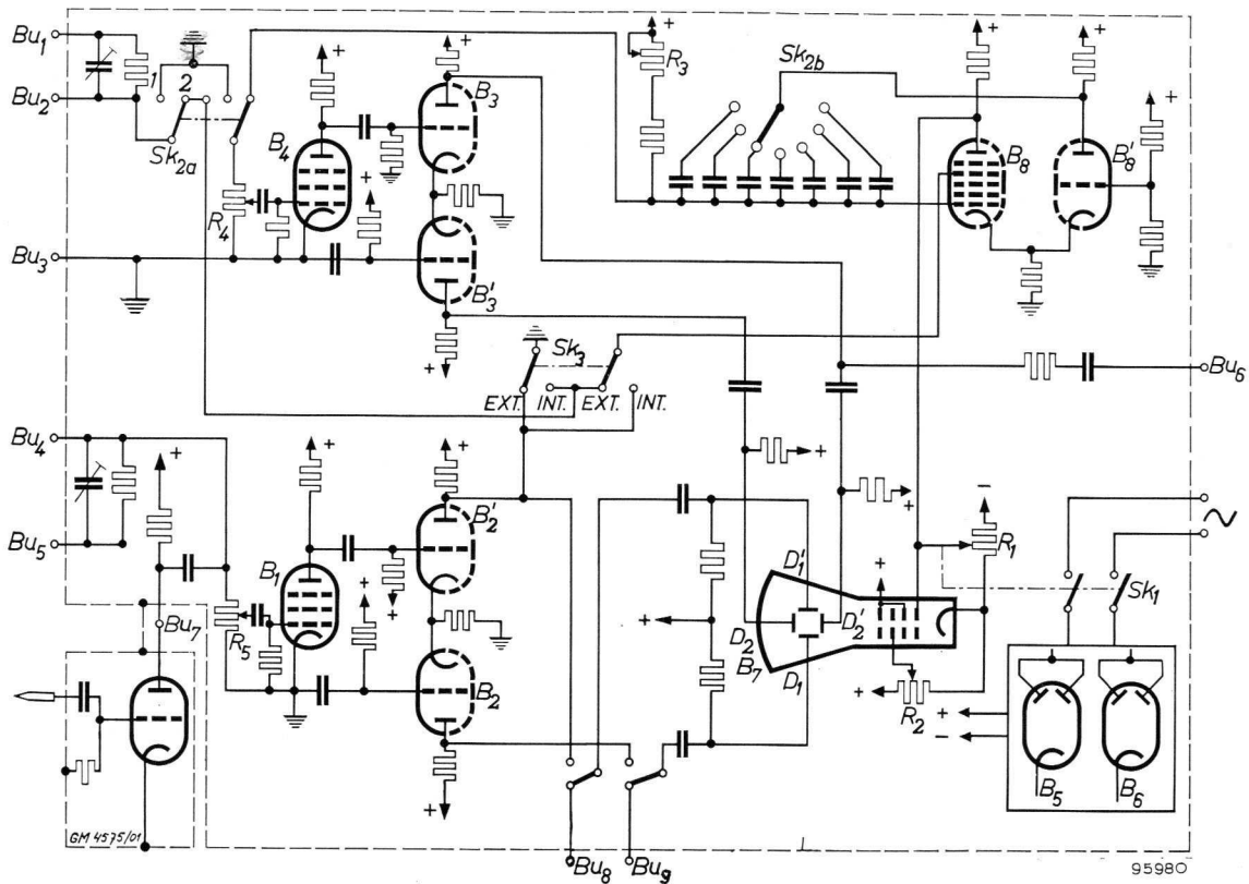
Fig. 2. Vereenvoudigd prinsieschema
