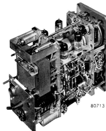
Fig. 1. Binnenaanzicht
