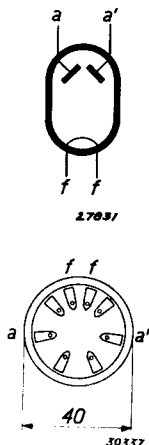
Abb. 2 Elektrodenanordnung und Socketanschlüsse.
