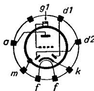
Sockelschaltschema
