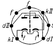
Sockelschalterschema
